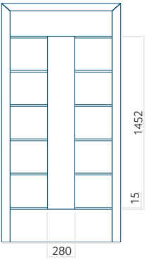
Dessin technique
